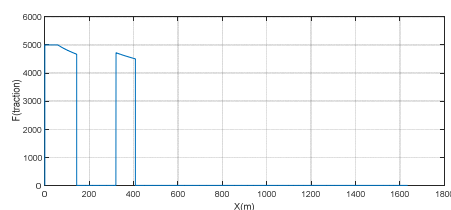
شکل ۱۳. نمودار نیروی کششی - مکان بهینه در سناریو ۵ فازی
