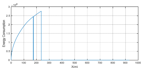
شکل ۲۱. نمودار انرژی - مکان بهینه در سناریو پنج‌فازی
