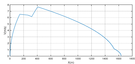
شکل ۱۲. نمودار سرعت - مکان بهینه در سناریو ۵ فازی
