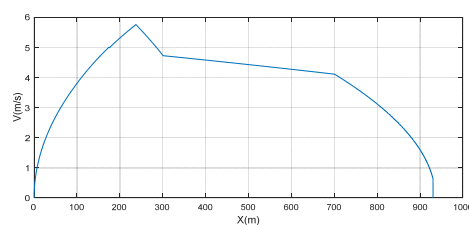
شکل ۱۹. نمودار سرعت - مکان بهینه در سناریو پنج‌فازی
