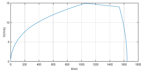
شکل ۵. نمودار سرعت - مکان تکرار اول در سناریو ۳ فازی
