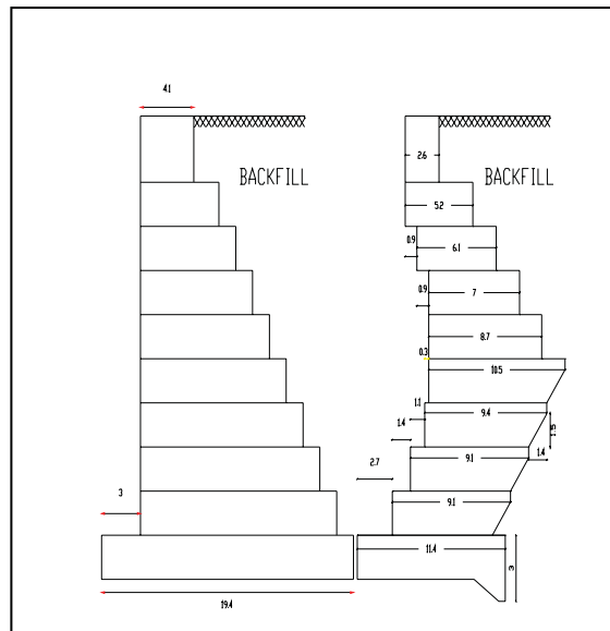
شکل ۸. مقطع بهینه درحالت‌های: مصالح پشت‌ریز با زاویه اصطکاک داخلی کمتر (شکل سمت راست)، ارتفاع متغیر بلوکها (شکل سمت چپ)
