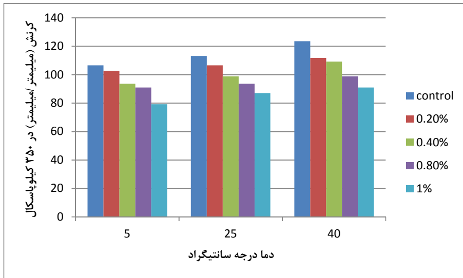
شکل ۷. کرنش نهایی کششی نسبت به دما
