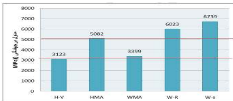
شکل ۱۱. تعیین MR برای نمونه‌های ساخته شده
