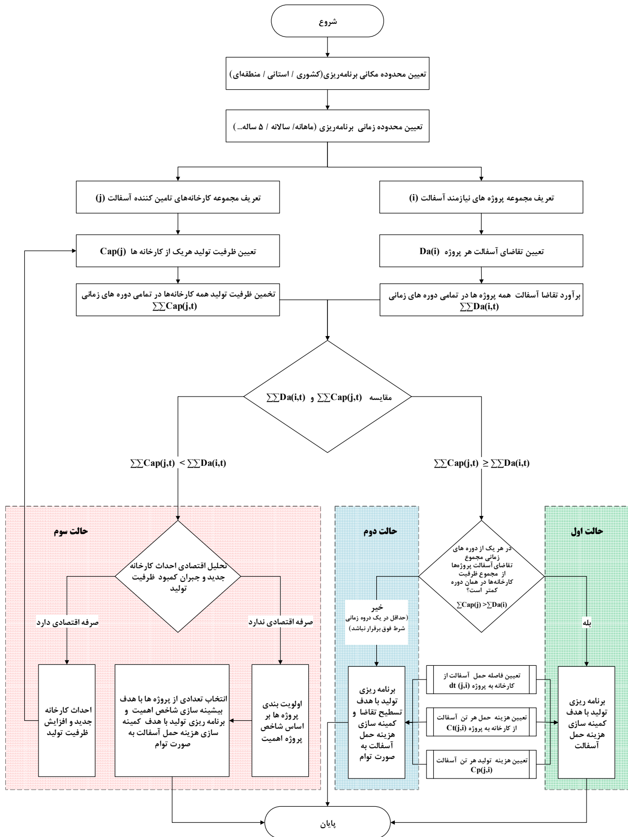
شکل ۴. مدل برنامه ریزی یکپارچه تولید و توزیع آسفالت (مدل بیتا)
