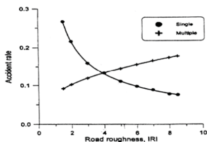
شکل ۱. رابطه بین نرخ تصادفات و ناهمواری روسازه [۹].
