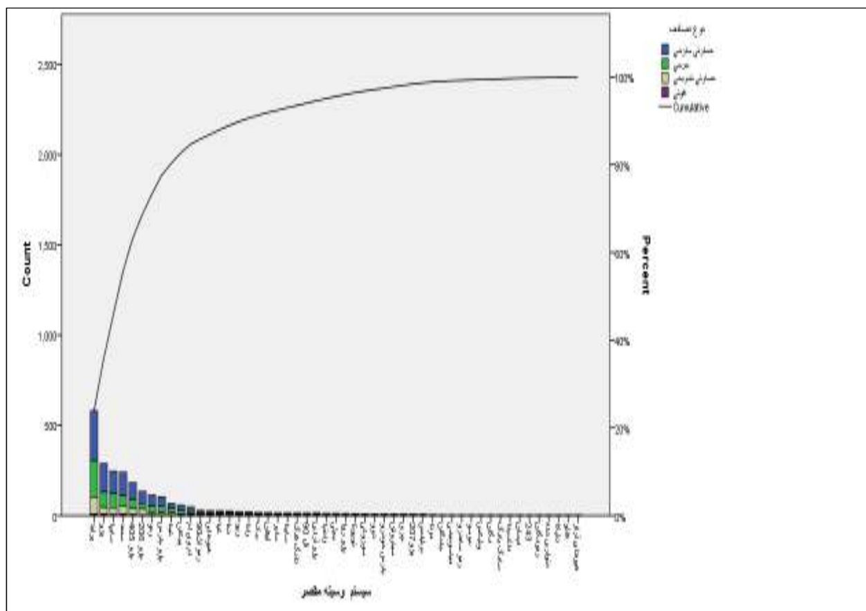
شکل ۳. نمودار پارتو تصادفات با توجه به سیستم وسیله مقصر
