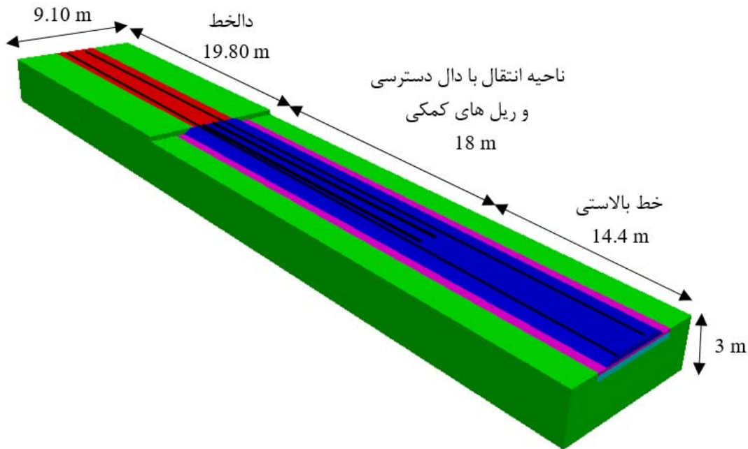
شکل ۱. مدل سه بعدی خط ریلی در محل ناحیه انتقال از داخل به خط بالاستی
