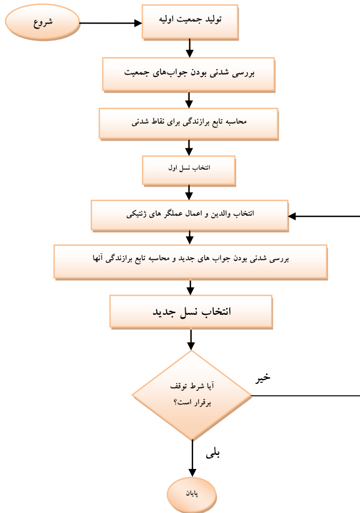
شکل 1. روندنمای الگوریتم ژنتیک پیشنهادی برای حل مسئله
