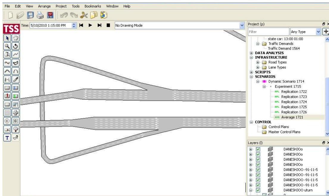
شکل 5. سناریو 2. ایجاد زیرگذر در محل دوربرگردان در محور کرمانشاه - بیستون
