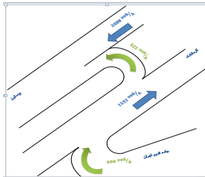
شکل 3. خلاصه برداشت حجم در محور کرمانشاه - بیسون
