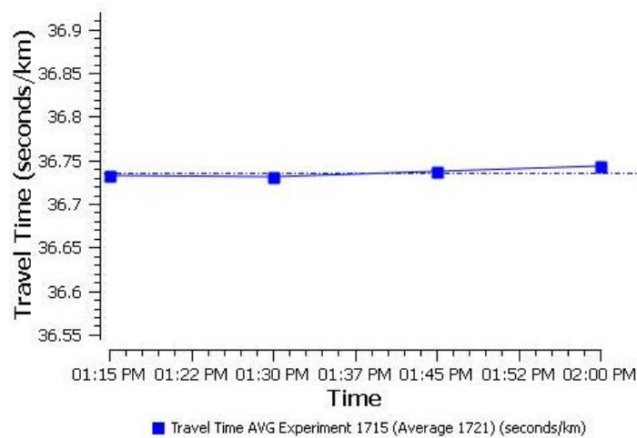
شکل 6. تأخیر در شبکه پس از اجرای سناریو 2 (بازه 15 دقیقه‌ای) در محور کرمانشاه - بیستون
