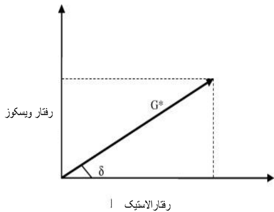
شکل 4. مولفه‌های مدول مختلط برشی
