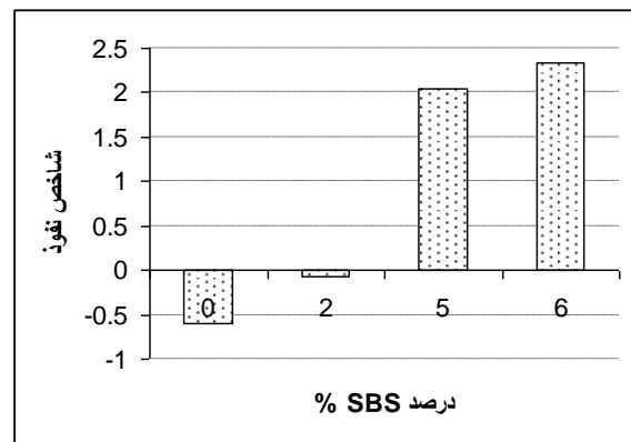
شکل 8. تغییرات شاخص نفوذ قیر با مقدار SBS
