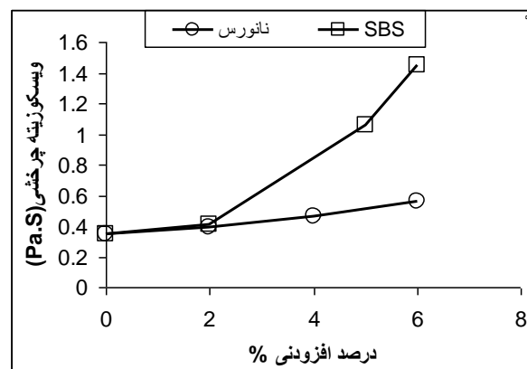
شکل 9. تغییرات ویسکوزیته دینامیکی با مقدار مواد افزودنی
