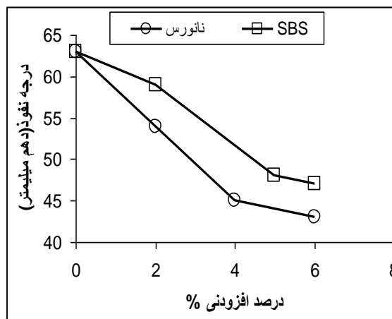
شکل 5. تغییرات درجه نفوذ با مقدار ماده افزودنی
