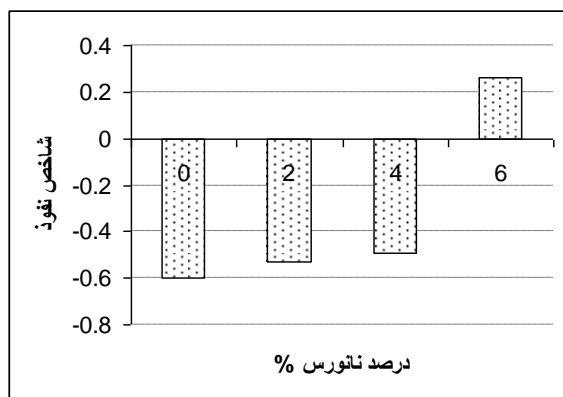
شکل 7. تغییرات شاخص نفوذ با درصد نانورس
