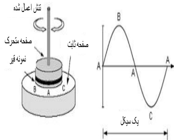
شکل 2. شماتیک آزمایش DSR
