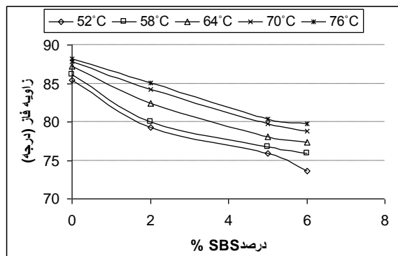
شکل 11. تغییرات زاویه فاز با مقدار ماده افزودنی SBS در
