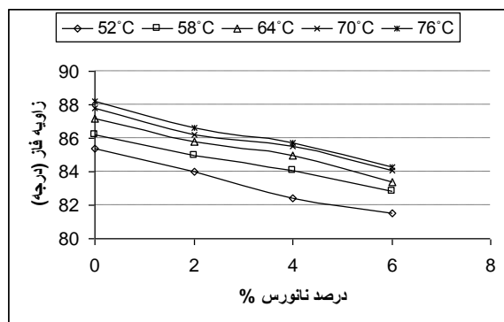
شکل 10. تغییرات زاویه فاز با مقدار ماده افزودنی نانو رس در دماهای مختلف
