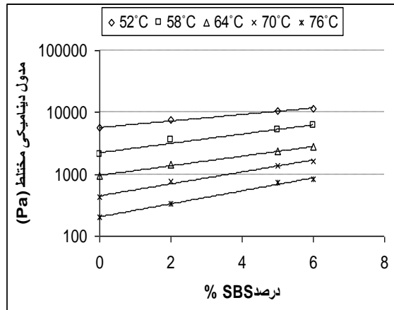
شکل 13. تغییرات مدول دینامیکی مختلط با مقدار ماده افزودنی SBS در دماهای مختلف
