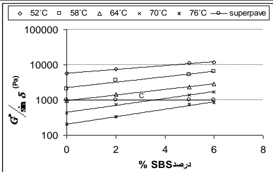
شکل 15. تغییرات شاخص G^*/\sin \delta با مقدار ماده افزودنی SBS
