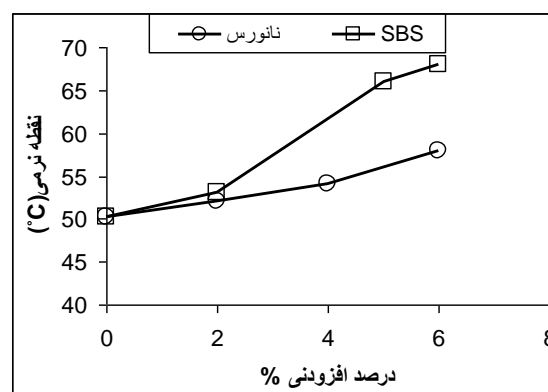
شکل 6. تغییرات نقطه نرمی قیر با مقدار ماده افزودنی
