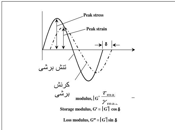
شکل 3. تنش و کرنش برشی در آزمایش DSR
