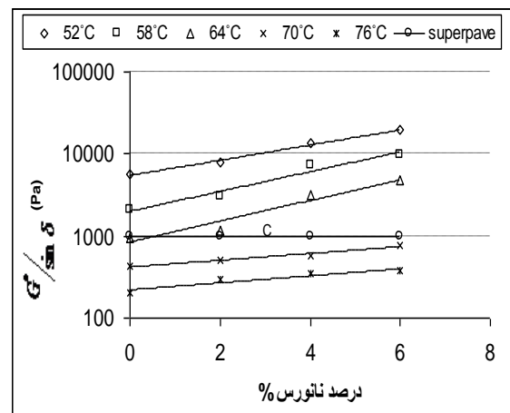
شکل 14. تغییرات شاخص G^*/\sin \delta با مقدار ماده افزودنی نانورس
