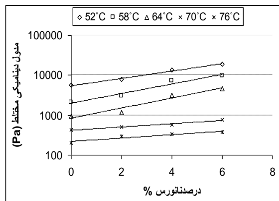
شکل 12. تغییرات مدول دینامیکی مختلط با مقدار ماده افزودنی نانورس در دماهای مختلف
