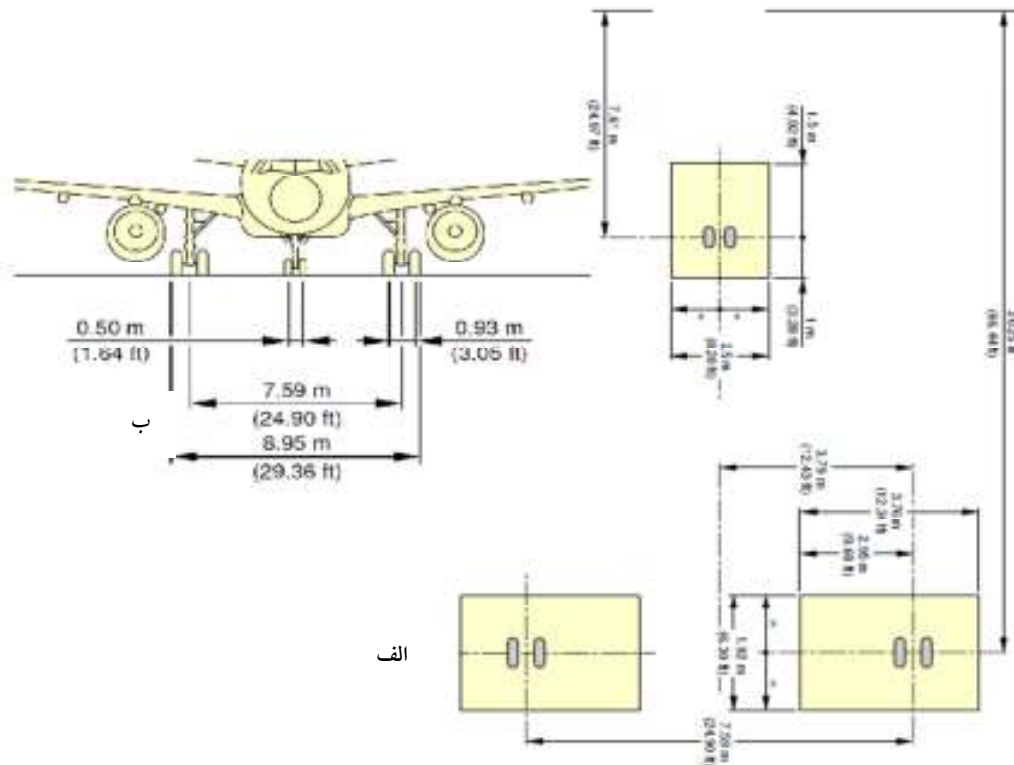
شکل ۳. الف. نحوه قرارگیری و فاصله چرخ‌های هواپیمای طرح Airbus,2014) A320 ب: نحوه قرارگیری و فاصله چرخ‌های هواپیمای طرح Airbus,2014) A320
