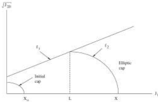
شکل ۲. مدل Cap
