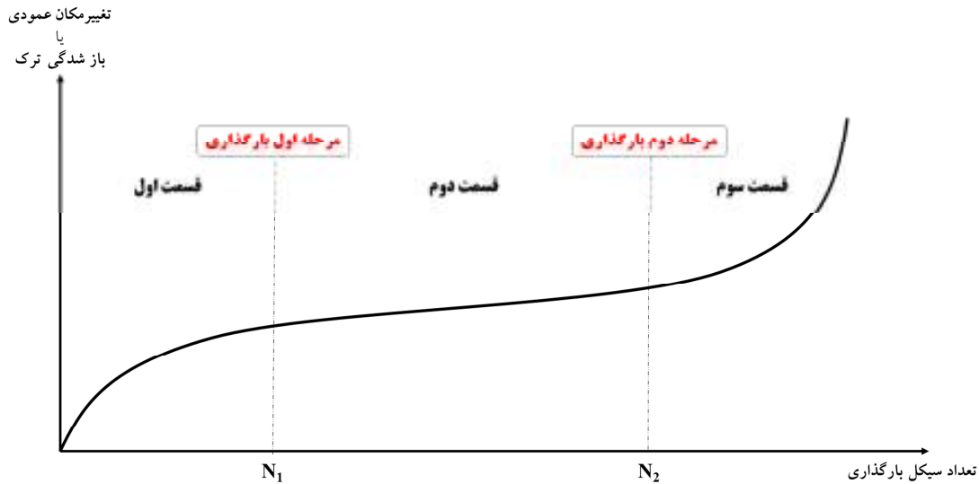
شکل ۶. نمودار سه قسمتی تغییر مکان در مقابل سیکل بارگذاری
