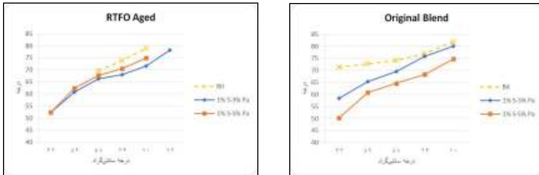
شکل ۱۳. زاویه فاز در دما و پیرشدگی‌های مختلفِ قیر حاوی ترکیب واکس پارافین و ساسوبیت
