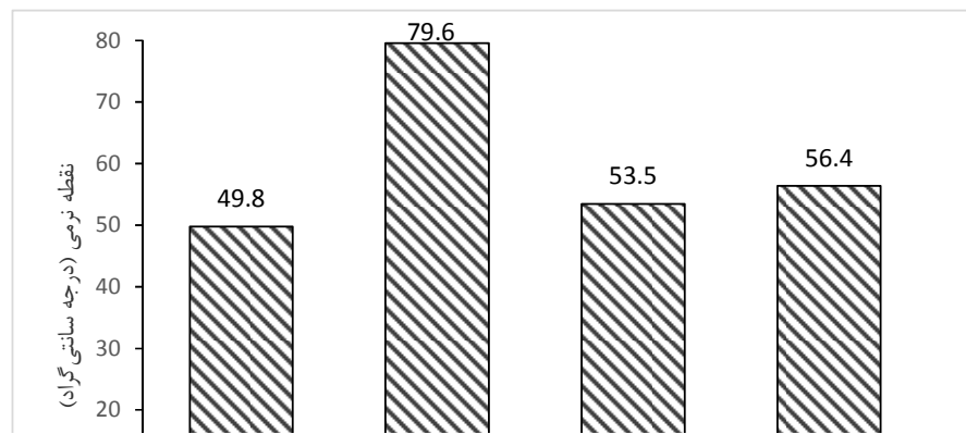
شکل ۲. تأثیر واکس‌های ساسویت و پارافین بر نقطه نرمی
