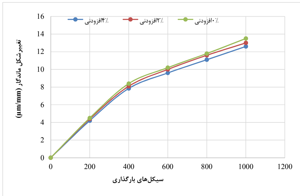
شکل ۷. تغییر شکل ماندگار در مقابل تعداد سیکل‌های بارگذاری سنگ‌دانه سیلیسی در دمای ۴۰ درجه سانتی‌گراد
