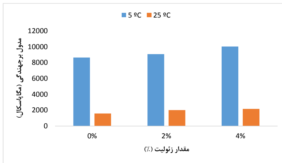
شکل ۴. مدول برجهندگی نمونه‌های با سنگ‌دانه آهک
