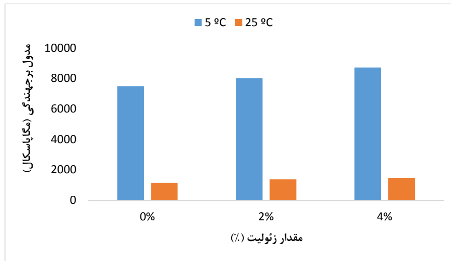
شکل ۳. مدول برجهندگی نمونه‌های با سنگ‌دانه سیلیسی
