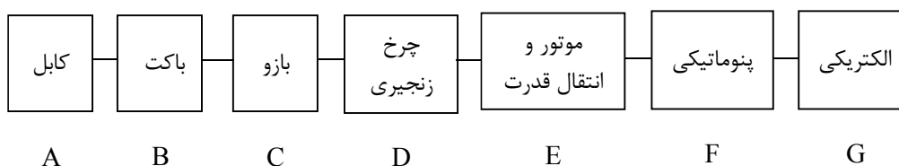
شکل ۳. دیاگرام بلوکی قابلیت اطمینان (RBD) شاول کابلی
