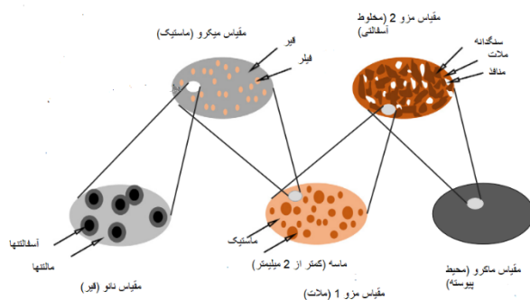
شکل ۱. مدل چند مقیاسی برای مخلوط‌های آسفالتی شامل مقیاس قیر، مقیاس ماسستیک (قیر و فیلر)، مقیاس ملات (ماسستیک و سنگدانه‌های ریزتر از ۲ میلیمتر)، مقیاس مخلوط (ملات و سنگدانه‌های درشت‌تر از ۲ میلیمتر) و مقیاس ماکرو (Yu et al., 2015)
